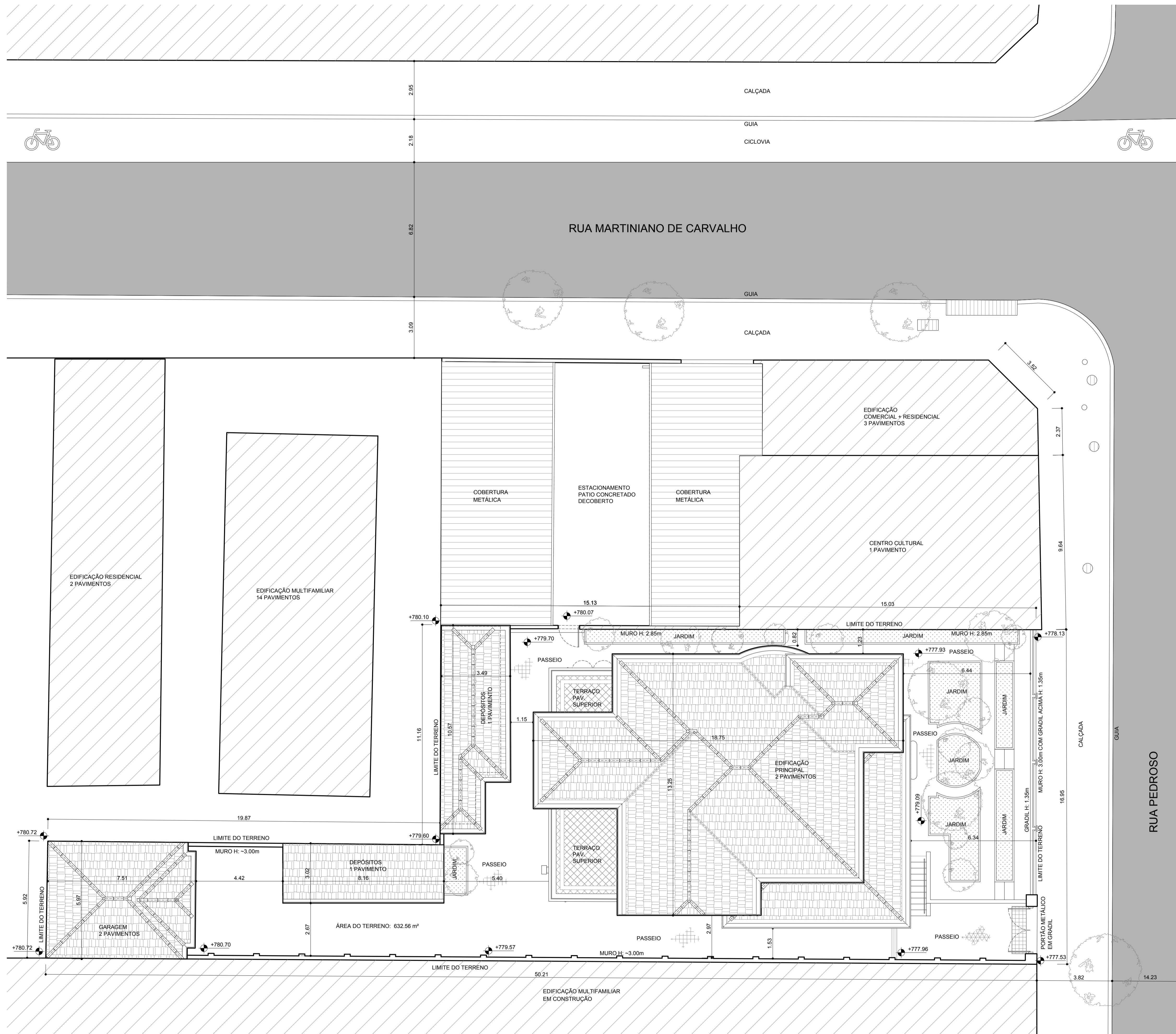
01 PLANTA DE LOCAÇÃO ESCALA 1:100
